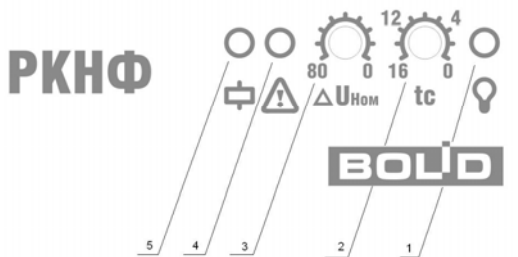
Рисунок 3. Лицевая панель РКНФ
