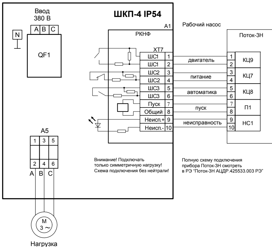
Рисунок 2. Схема электрическая подключения шкафа при эксплуатации
