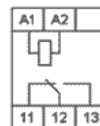
СХЕМА ВКЛЮЧЕНИЯ
