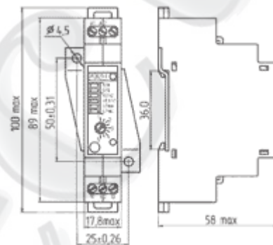
реле с креплением винтами
