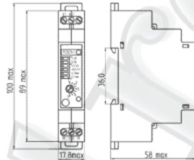
реле с креплением на DIN-рейку
