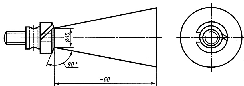
Рисунок 1 — Коническая оправка
